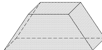
UPCHÁVKA VLNY TRAPÉZOVÉHO PLECHU Z MINERÁLNEJ VLNY
