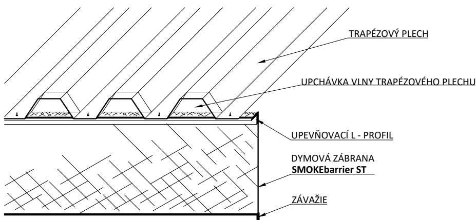
UPCHÁVKA VLNY TRAPÉZOVÉHO PLECHU Z MINERÁLNEJ VLNY
